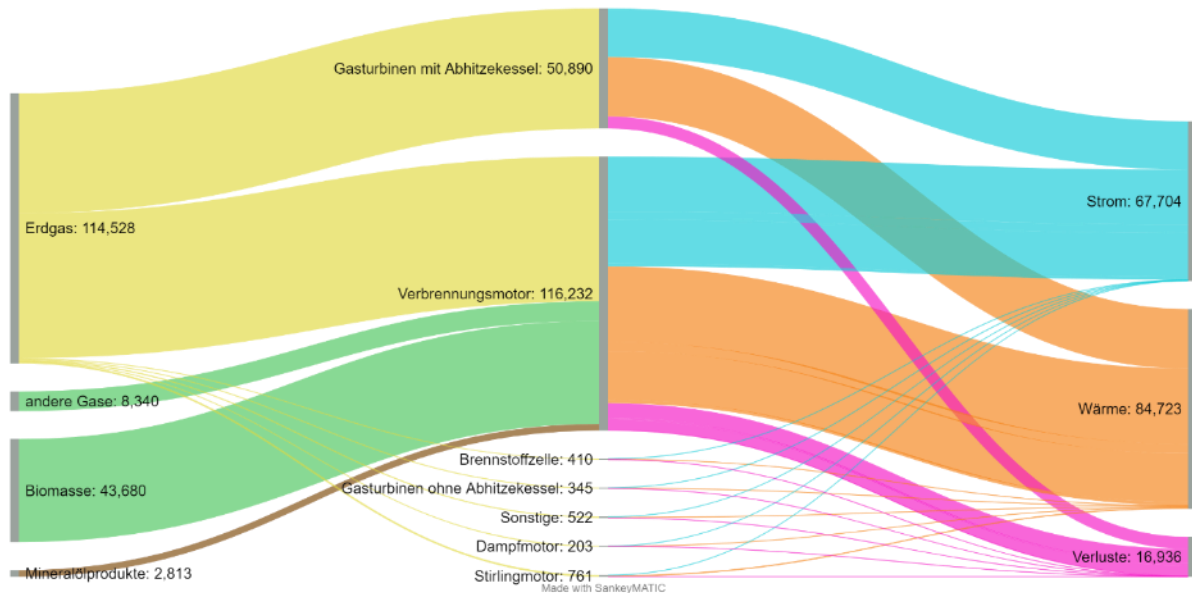
Abbildung 27 Energieflussdiagramm der Kraft-Wärme-Kopplung
